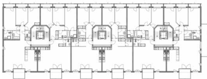
Plans d'étage type
